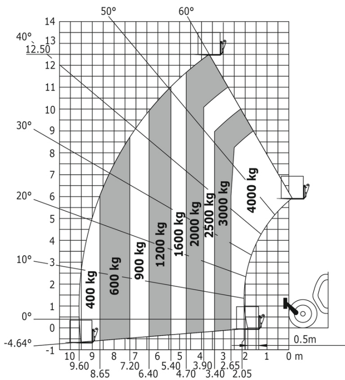
Maschine auf Rädern mit Gabelzinken - mit Niveaueausgleich
